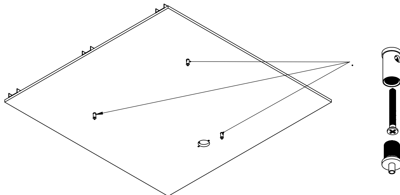
(1) Preparar o forro e fixar os acessórios de fixação.
