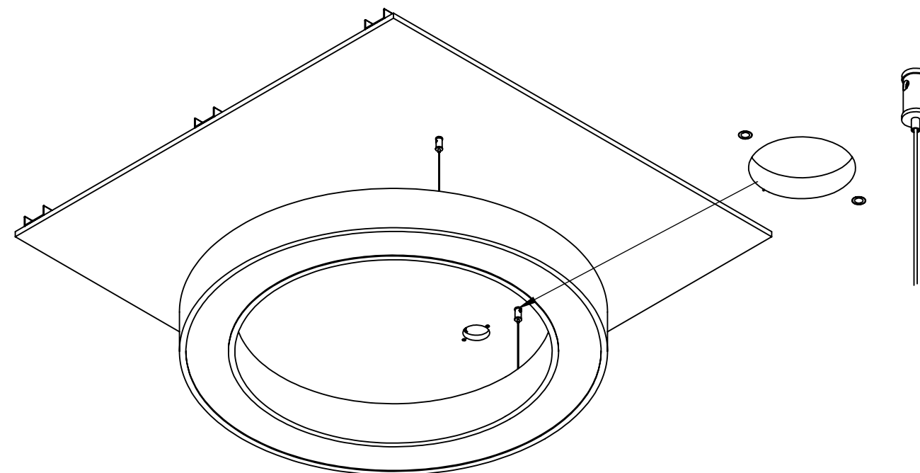
(2) Posicionar a luminária no local e ajustar altura.
