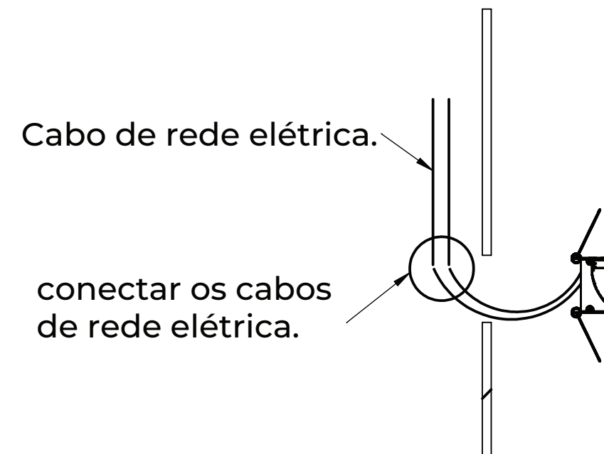
2. Conecte os cabos de rede.
