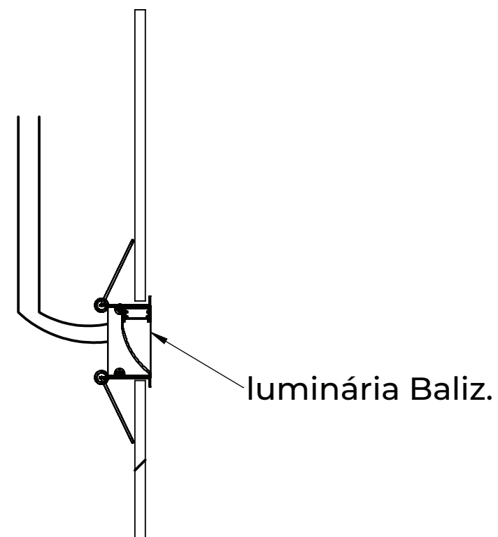
4. Luminaria Baliz já instalada na superfície.
