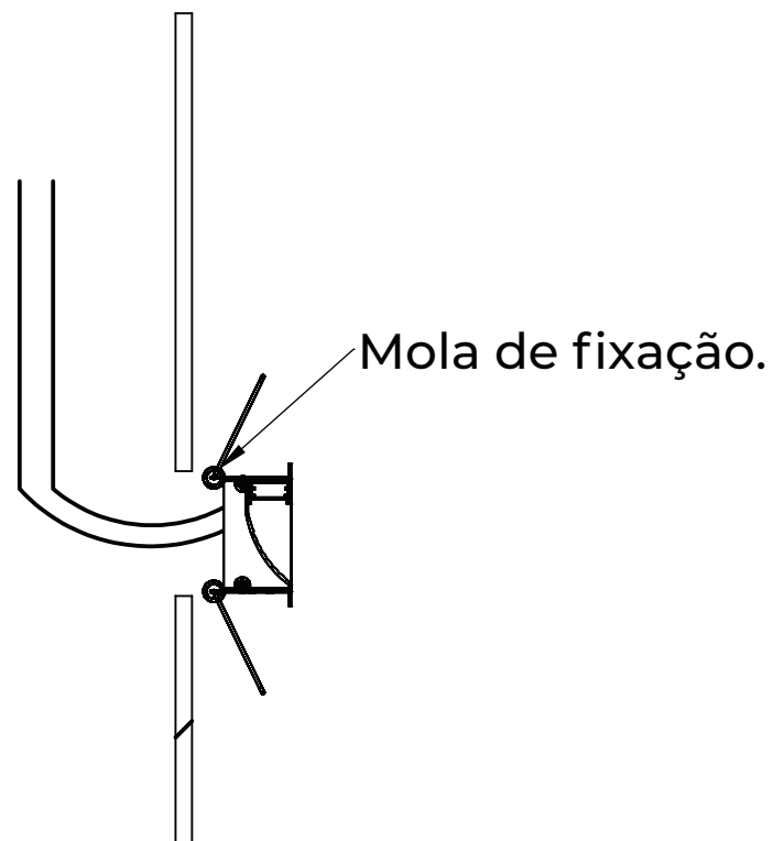
3. Suspenda a luminária pressionando as molas para encaixe.
