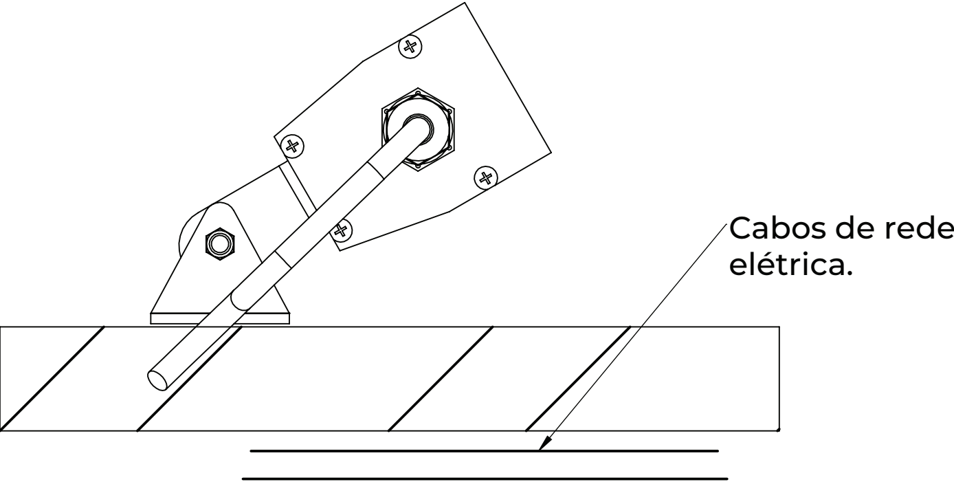
3. Conecte os cabos de rede elétrica.
