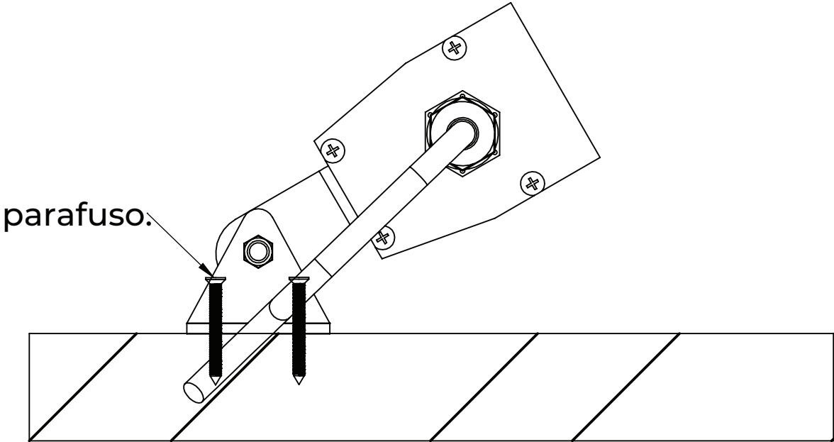
2. Trave o suporte de fixação da luminária usando os parafusos.
