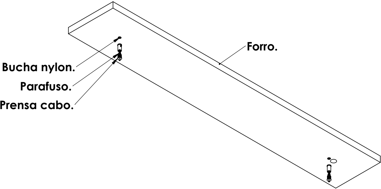
1. Fure a superfície demarcada e encaixe as buchas nylon e prensa cabo.
