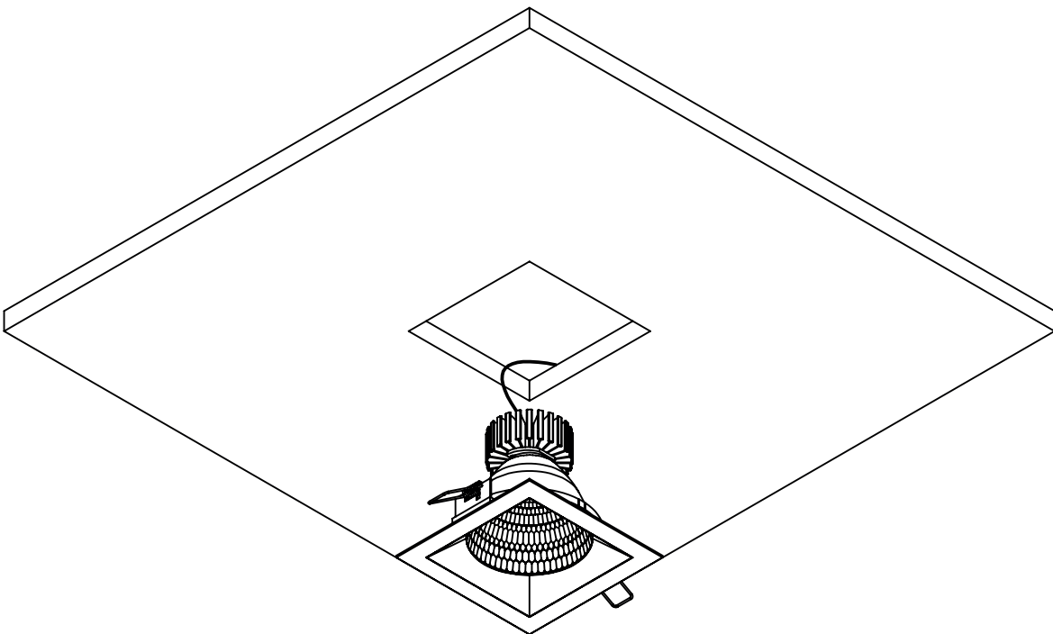
3. Posicione o driver sobre o forro e encaixe a luminária no forro.
