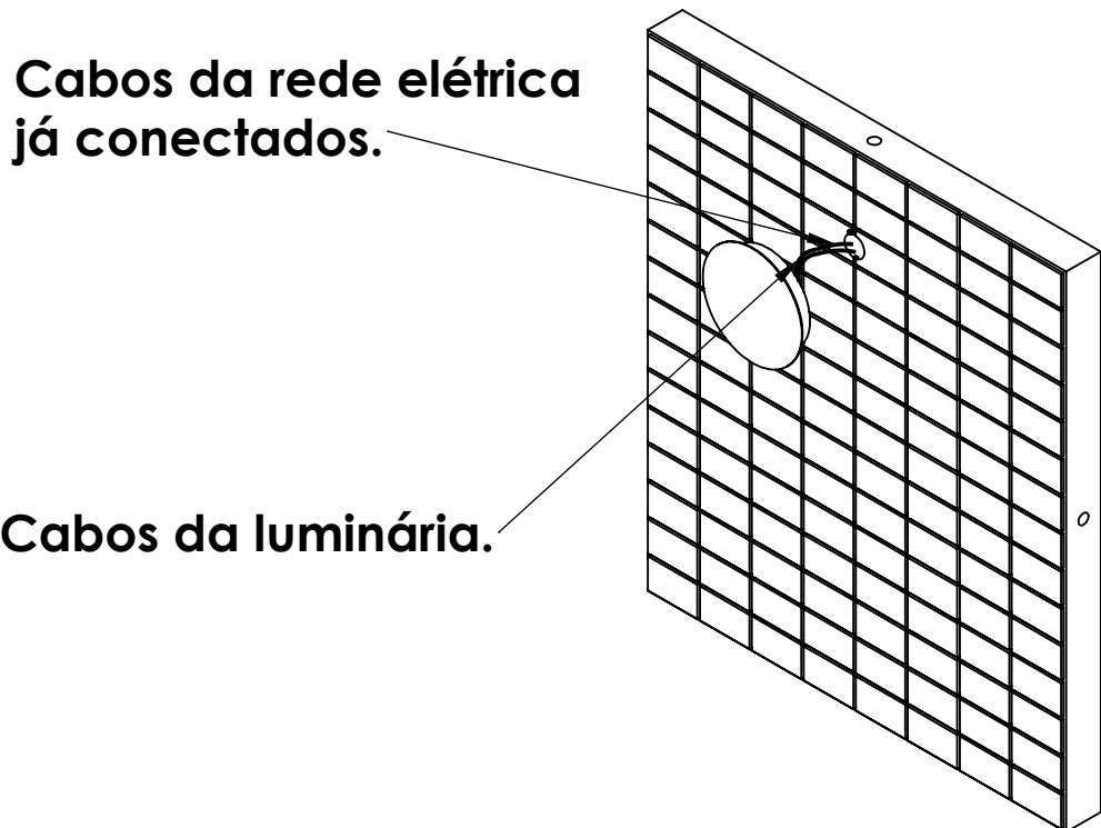
3. Suspenda a luminária e fixe junto ao parafuso.
