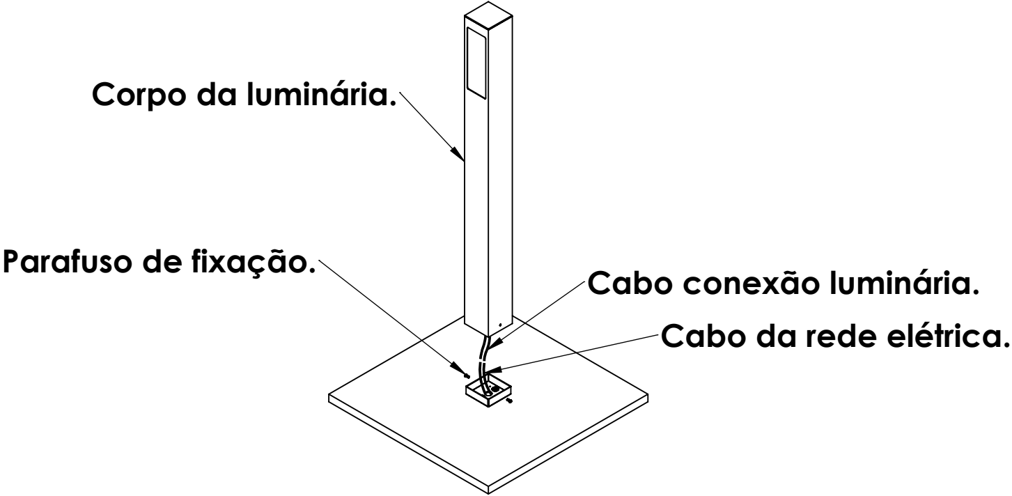
2. Conecte os cabos da luminária na rede elétrica e fixe a luminaria com parafusos.
